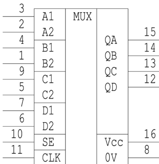
Рис. 1. Условное графическое обозначение микросхем 1564КП13 ЭП.
