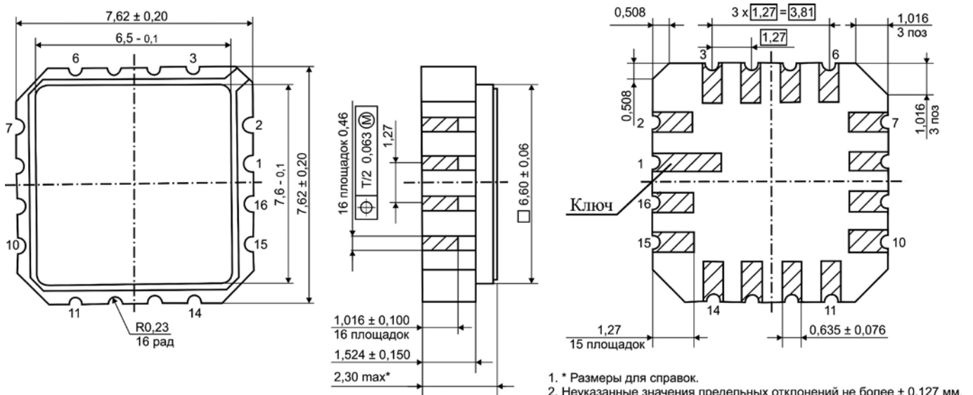
Рис. 4. Корпус 5119.16-А
