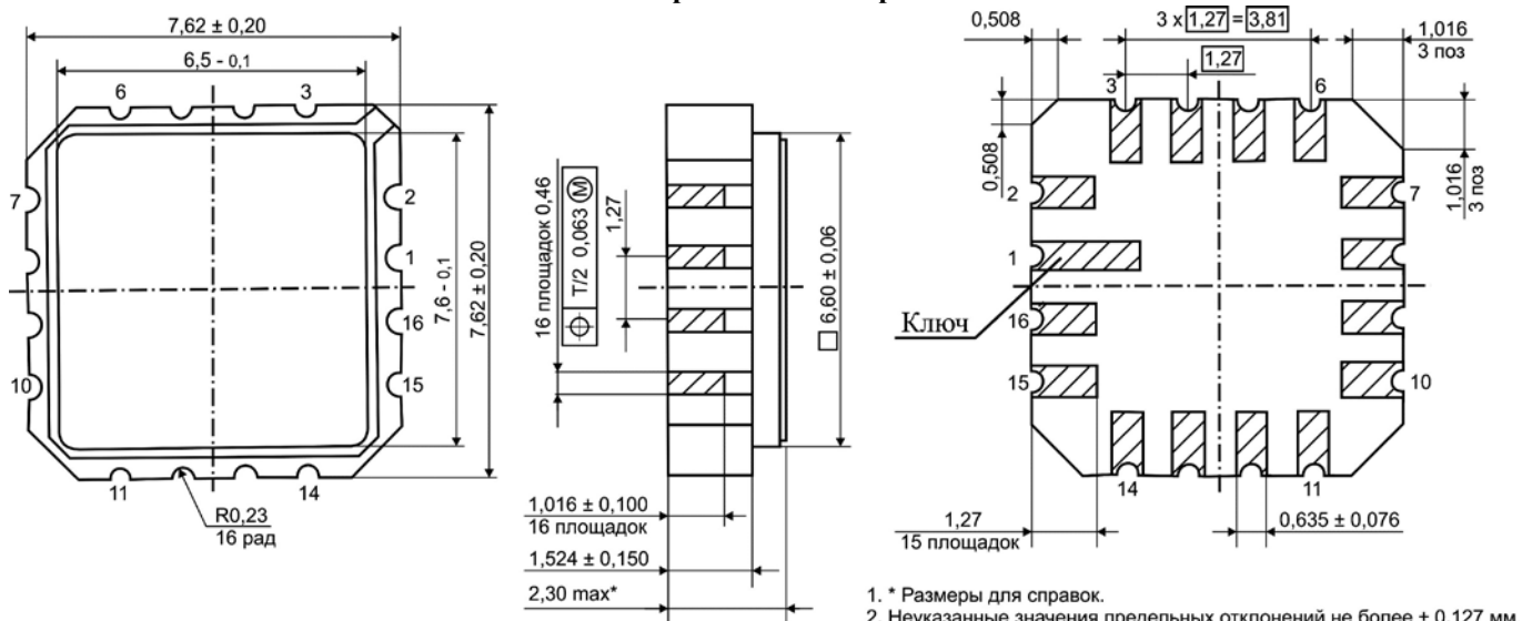
Рис. 7. Корпус 5119.16-А Размеры в миллиметрах.
