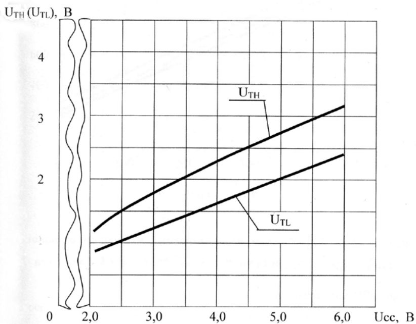
Рис. 5. Типовые зависимости порогового напряжения низкого (высокого) уровня от напряжения питания при t = +125\text{ }^{\circ}\text{C} для микросхем 1564ТЛ2 ЭП.
