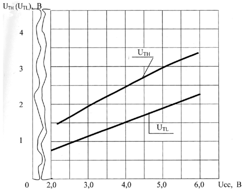
Рис. 3. Типовые зависимости порогового напряжения низкого (высокого) уровня от напряжения питания при t = 25\text{ }^{\circ}\text{C} для микросхем 1564ТЛ2 ЭП.
