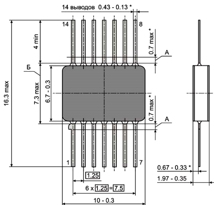
Рис. 6. Корпус 401.14-5 Размеры в миллиметрах.
