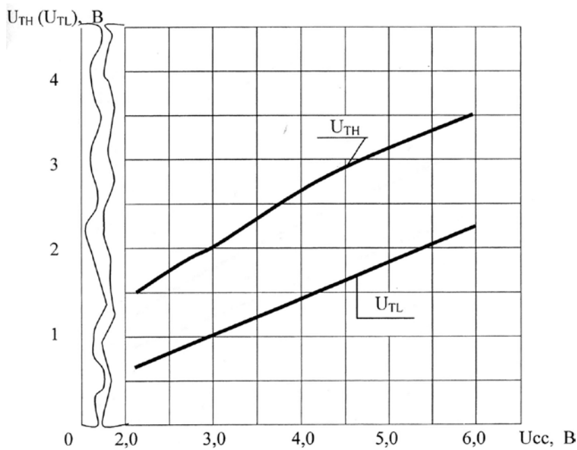
Рис. 4. Типовые зависимости порогового напряжения низкого (высокого) уровня от напряжения питания при t = -60\text{ }^{\circ}\text{C} для микросхем 1564ТЛ2 ЭП.
