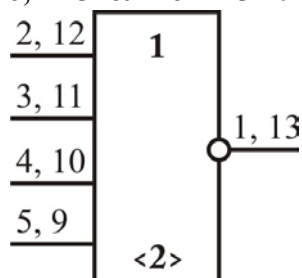
Т а б л и ц а 2. Таблица назначения выводов микросхем 1526ЛЕ6, Б1526ЛЕ6 – 1ЭП.
