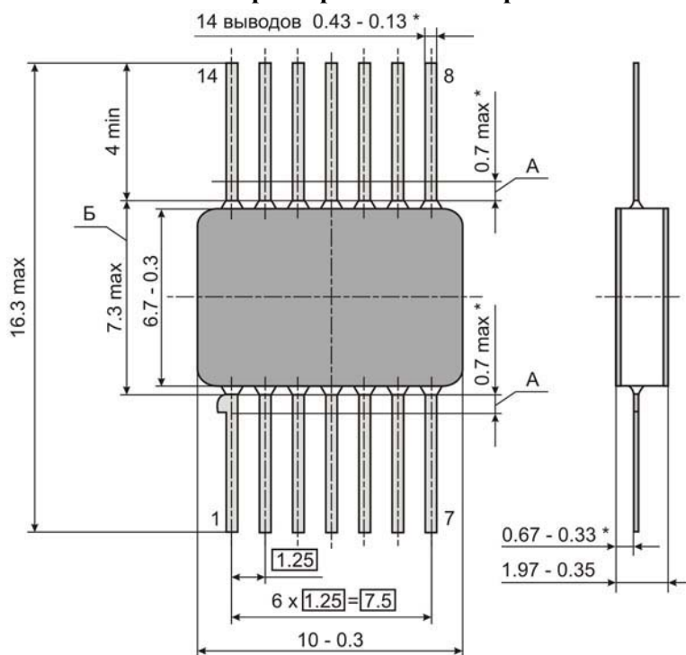
Рис. 2. Корпус 401.14-5 размеры в миллиметрах.
