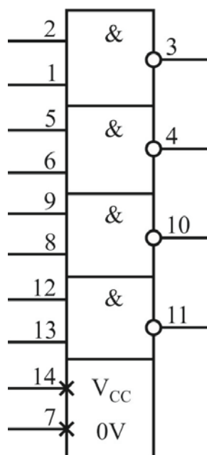
Рис. 1. Условное графическое обозначение микросхем 564ЛА7 ЭП.
