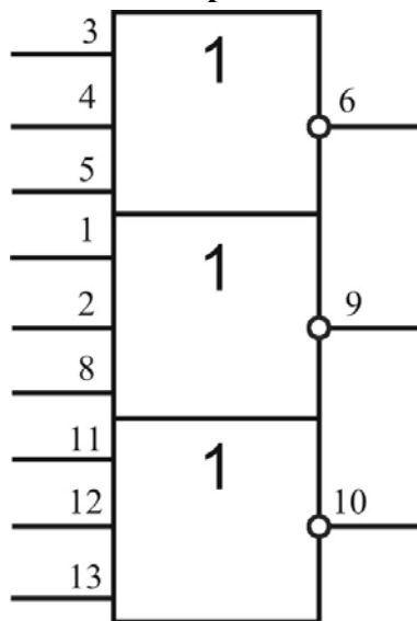
Рис. 1. Условное графическое обозначение микросхем 564ЛЕ10В.
