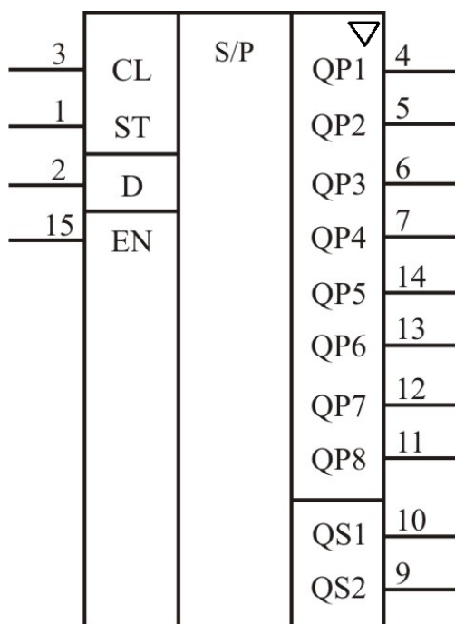
Рис. 1. Условное графическое обозначение микросхем 564ПР1В.
